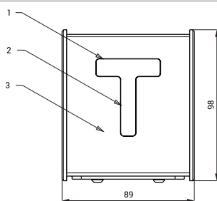
SLZA 30A
